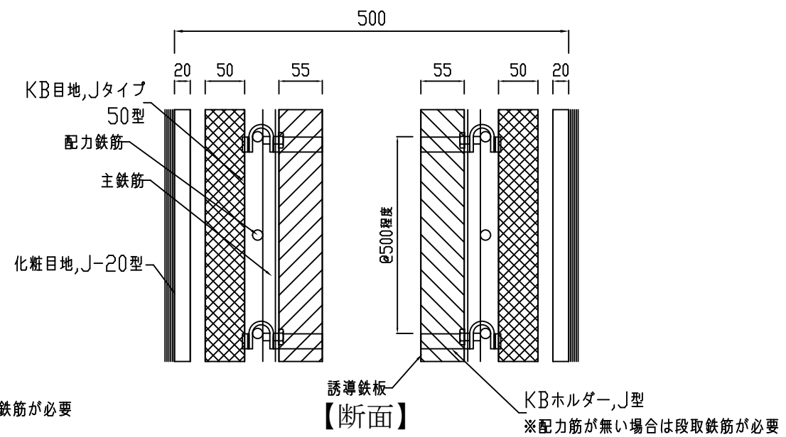
詳細図 Jタイプ50型
