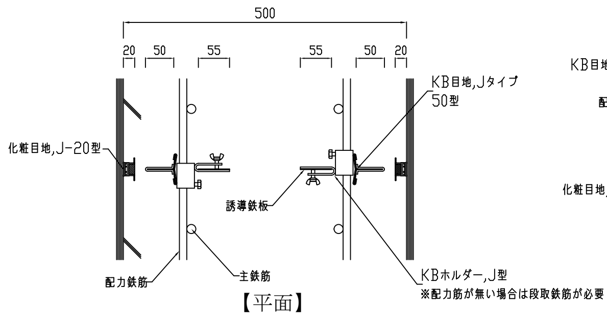
詳細図 Jタイプ50型
