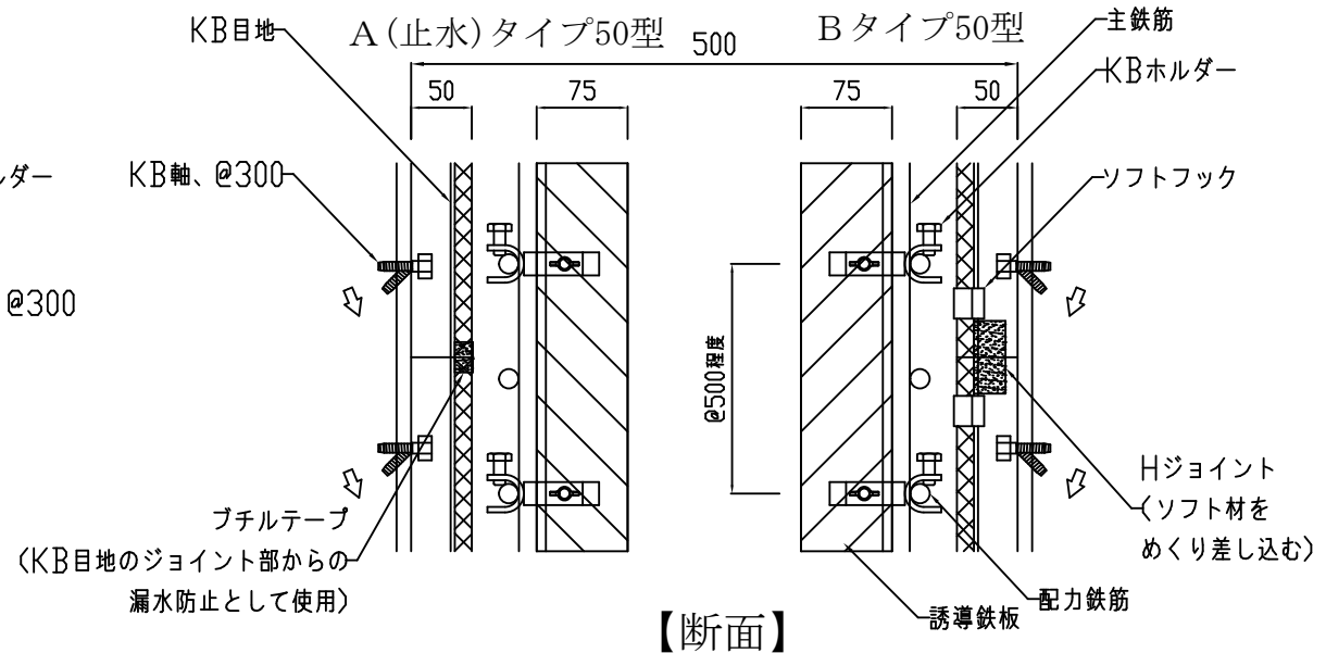
詳細図
