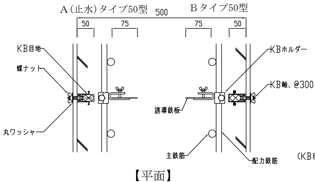
詳細図
