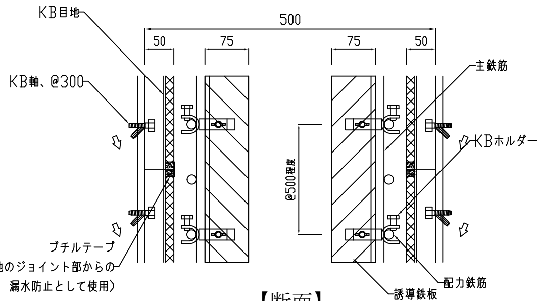
【断面】
